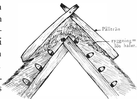
5. Ryggnigen, schema.
