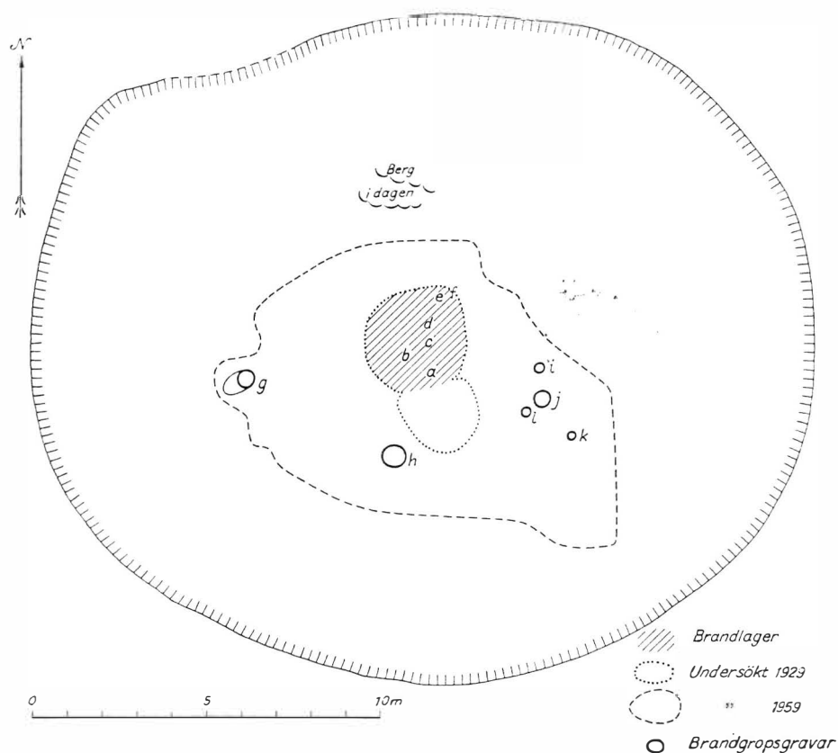
Fig. 1. Plan över rösebotten i Tärby Stommen.
