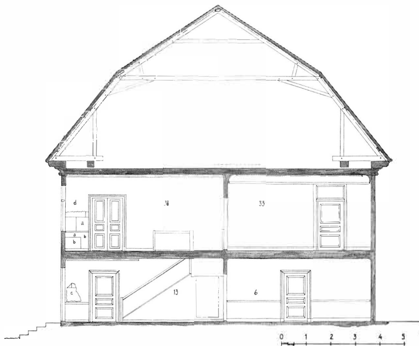
Sektion genom förstugorna mot öster. Vindfång inom rum 13 ej inritat. Uppmätning Iwar Andersson 1963.
