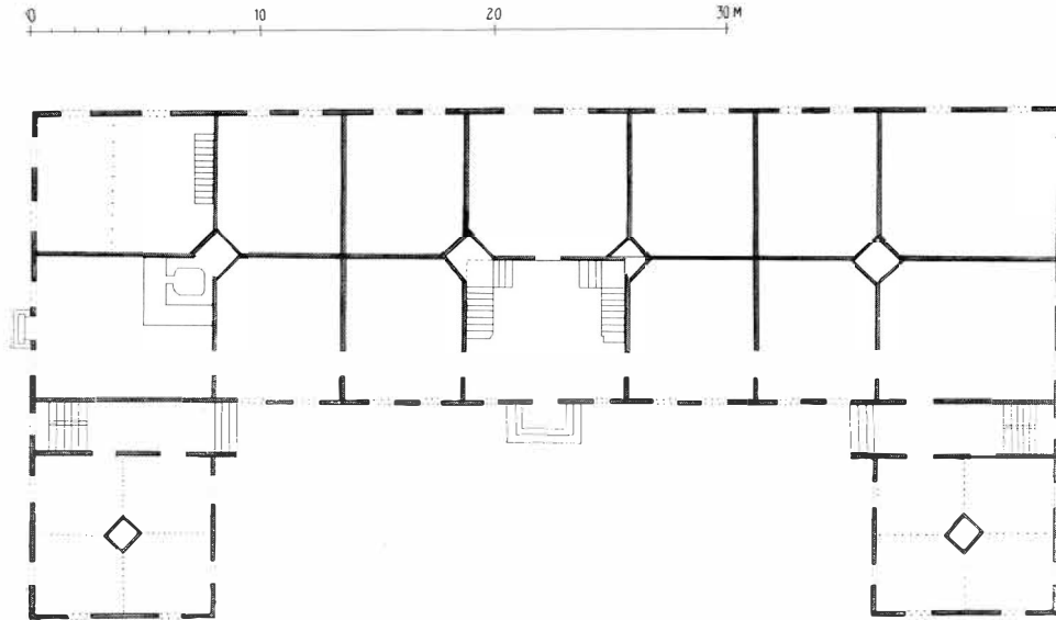
”Undre våningen”. Omritning av äldre plan förvarad i Göteborgs landsarkiv. Originalets alnmått förvandlade till meterskala.
