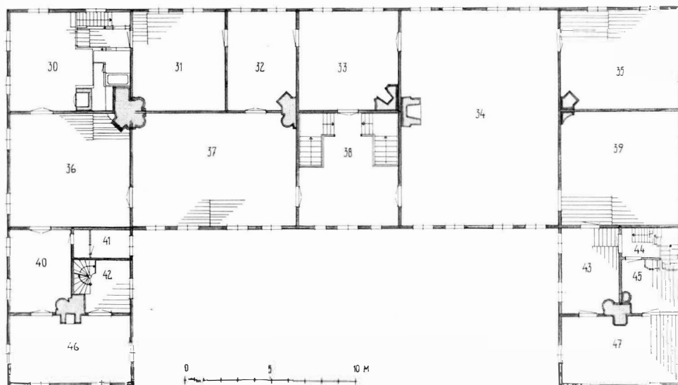
Torpa, plan av bottenvåningen (överst) och övre våningen. Uppmätning av Ivar Andersson 1963.
