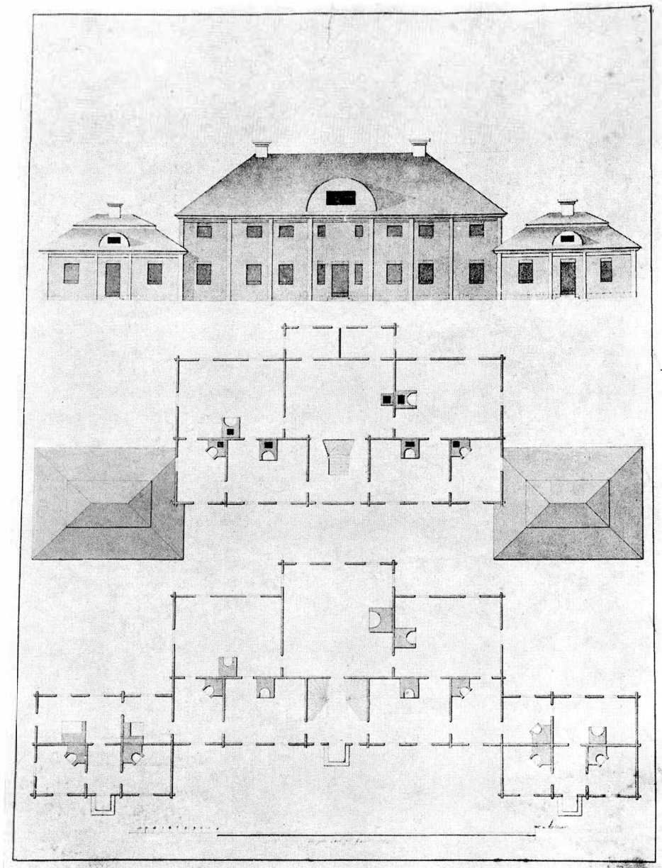
4. Fasadritning och plan av Torpa corps de logis. Ritningen daterad 1777.
