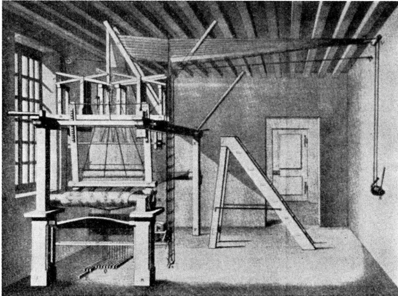
Zampelvävstol för bildvävnad. (1750)
