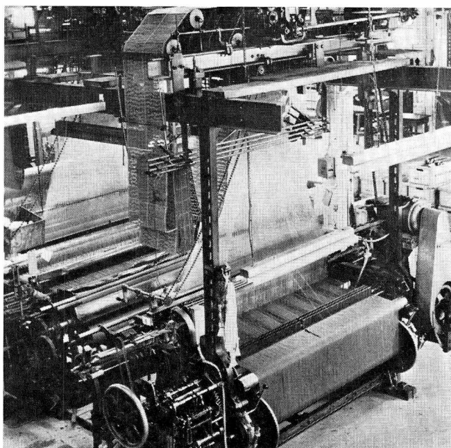
Mekanisk vävstol med jacquardmaskin.
