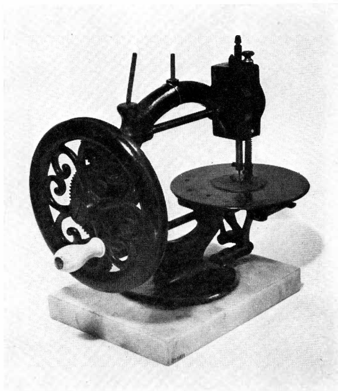
Symaskin, handdriven, entrådlig. Maskinen inköptes i London av L. G. Wingqvist, Fritsla, för hustrun Lovisas räkning. Märkt: R. M. Eantzer & Co. Patentees & Manuf Hamilton Canada West. Time Utilizer Trade mark No 131656. Patented in America Grt Britain and the Continent. May 16 & June 17 1867. BM 51.874.
