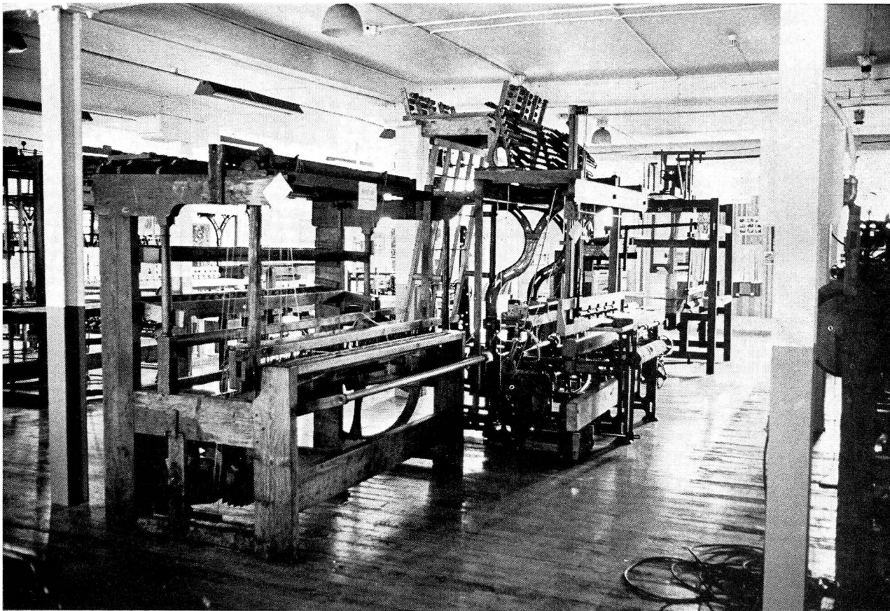
Textilindustrimuseet öppnat 21 maj 1972. Några av vävstolarna.
