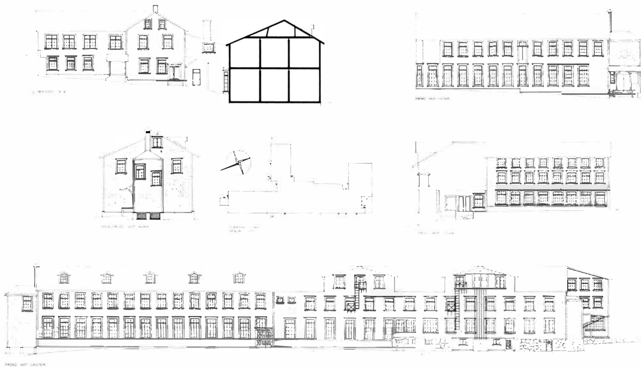
A. J. BORGS VÄVERI AB, gamla fabriken, Harpebo. Fasader, sektion. Uppmätning juni 1972.
