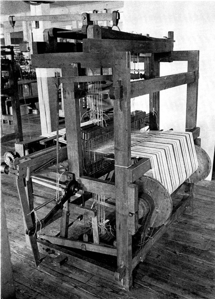
Textilindustrimuseet. Enkel jacquardväv för hemvävnad. Konstruerad av Fritz Sterner, Överlida.
