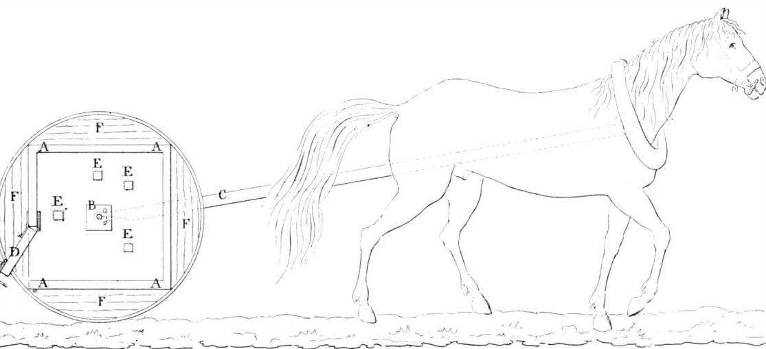
Teckning ur C G Rydins skrift "Gjutna kalkbrukshus" från 1834. Rydins "betongblandare" — efter en runda på Stora torget var murbruket färdigblandat.
