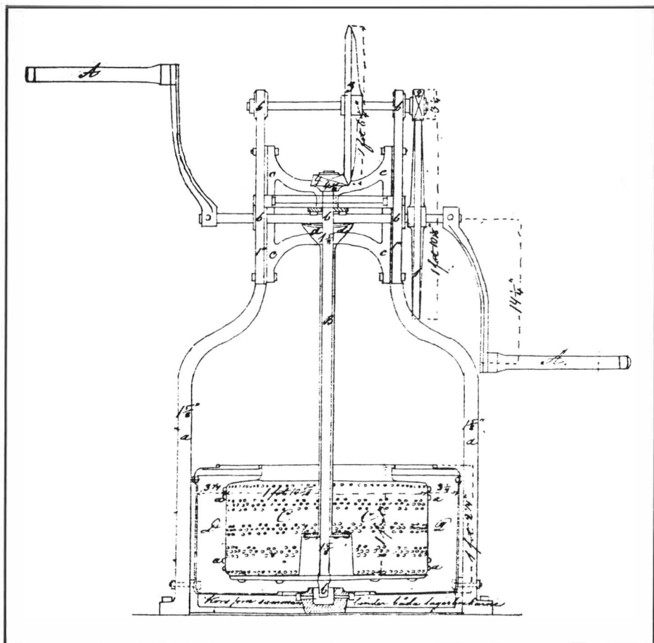
Patenterad torkningsmaskin av typ använd vid Lydde. AP 1850.
