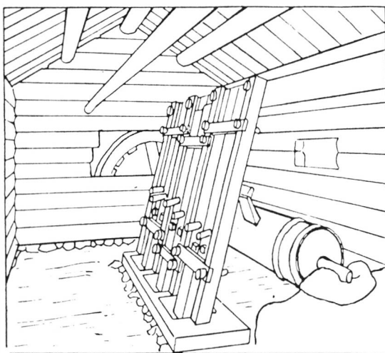
Interiör av vadmalsstamp från Älvdalen. Teckning U. Rothman i Ull och Ylle.
