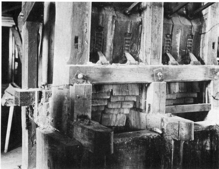
Stamp med fyra stötars hos Scheele i Alvesta. GHM.
