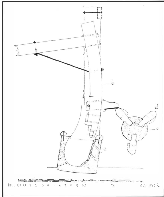
Sektion av stamp i Barevad Skåne: a-hjulaxel, b-stamp, c-kum d-hävarm. C.A. Althin i Kulturen 1936.
